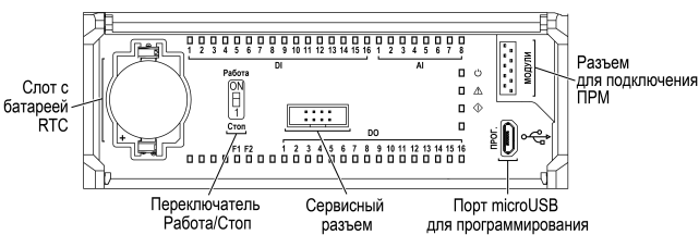
Рисунок 9 – Лицевая панель под крышкой
