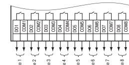
Рисунок 4 – Схема подключения нагрузок к ВЭ типа «Р»
