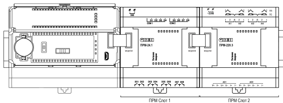
Рисунок 7 – Расположение модулей расширения на шине
