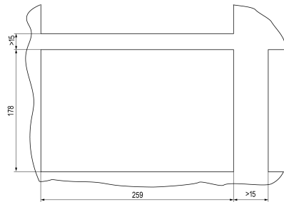
Рисунок 2 – Установочные размеры прибора
