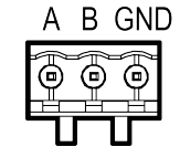
Рисунок 5 – Назначение контактов разъема RS-485-3
