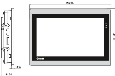
Рисунок 1 – Габаритные размеры прибора
