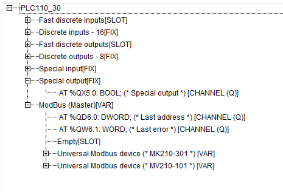
Рис. 3.3.7. Подэлементы Universal Modbus Device в конфигурации ПЛК
