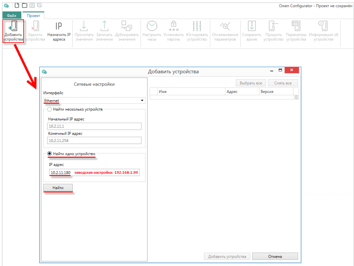
Рис. 2.3. Настройки подключения по интерфейсу Ethernet для модуля с заводскими настройками
