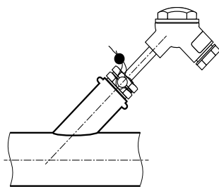
Рисунок 5.4 – Пломбировка КДТС045 (КДТС145, КДТС035)
