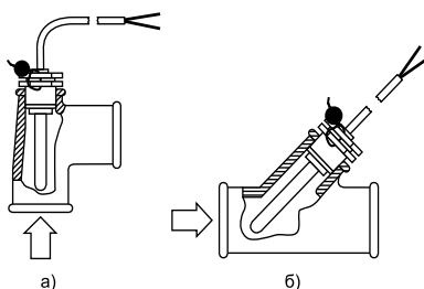
Рисунок 5.2 – Пломбировка КДТС054
