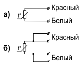
Рисунок В.1 – Схема подключения КДТС с кабельными выводами: а) двухпроводная схема, б) четырехпроводная схема
