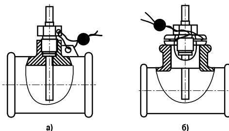
Рисунок 5.5 – Пример пломбировки КДТС054 прямого погружения
