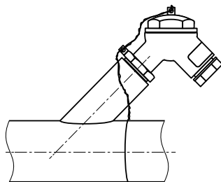
Рисунок 5.1 – Пломбировка КДТС105
