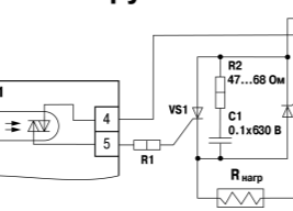
Рисунок 14 – Управление двумя тиристорами, подключенными встречно-параллельно
