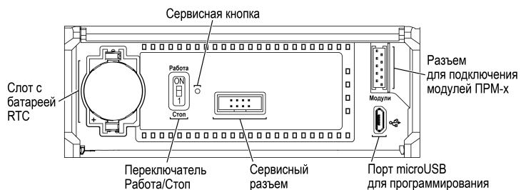
Рисунок 16 – Лицевая панель под крышкой
