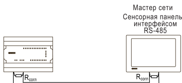
Рисунок 11 – Типовая схема подключения в режиме Slave
