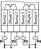
Рисунок 10 – Схема подключения нагрузок типа «КТ»
