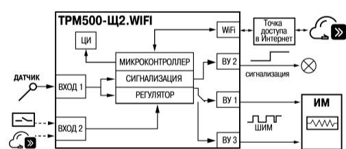
Рисунок 4 – Функциональная схема прибора
