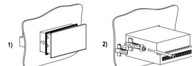
Рисунок 2 – Монтаж прибора щитового крепления
