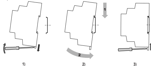
Рисунок 1 – Установка прибора
